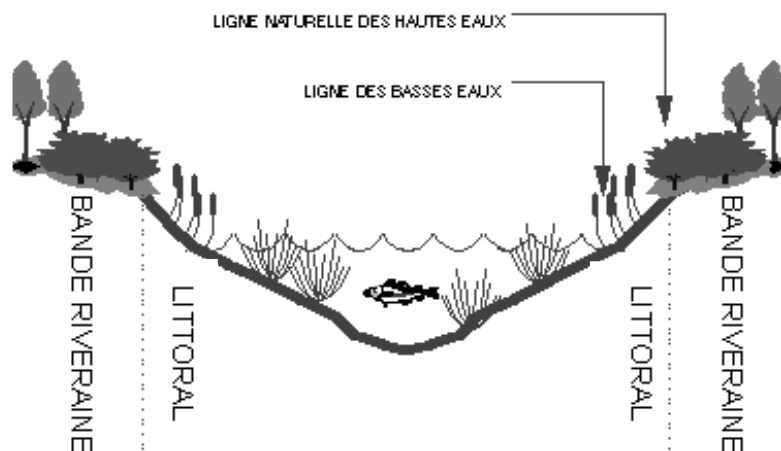
Figure 2.7b : Ligne naturelle des hautes eaux
