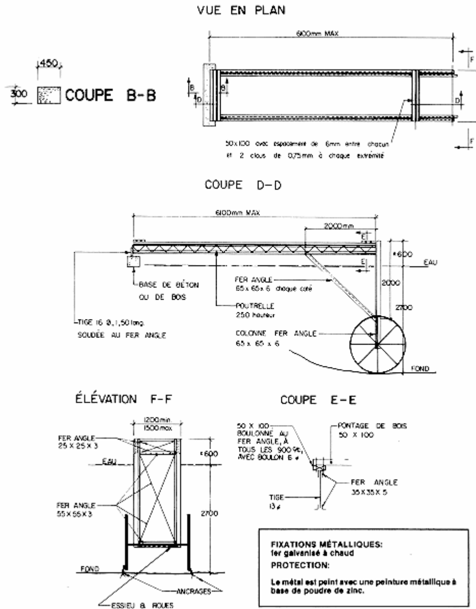
Figure 9.3.4b : Embarcadère amovible roulant, construit sur place
